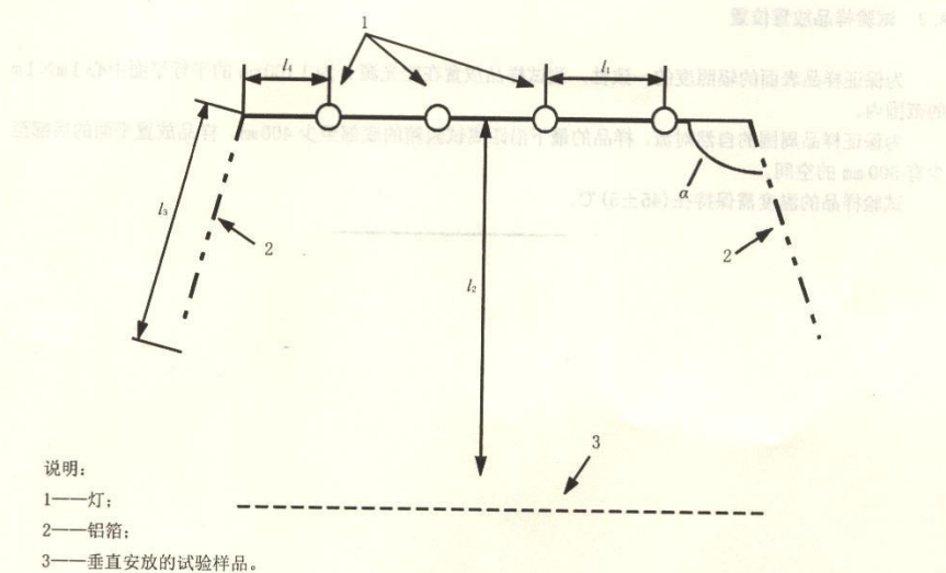
图A.1 光源布置示意图(俯视图)
