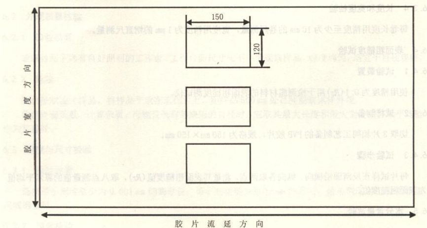
图2 热收缩试验试样剪取示意图
