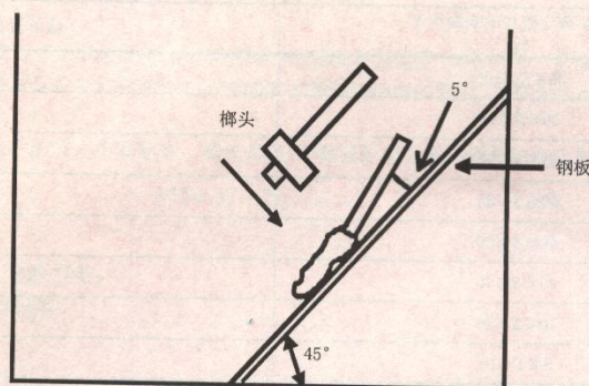
图3 敲击试验箱示意图
